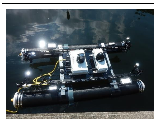
調査・点検用水上スライダー Hy-CaT （桁下点検用ユニット装備）
